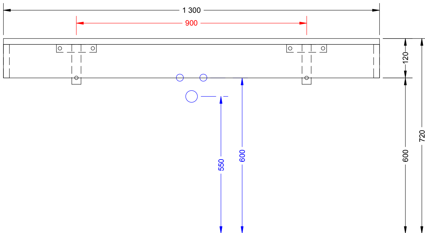
PŘEDNÍ POHLED
