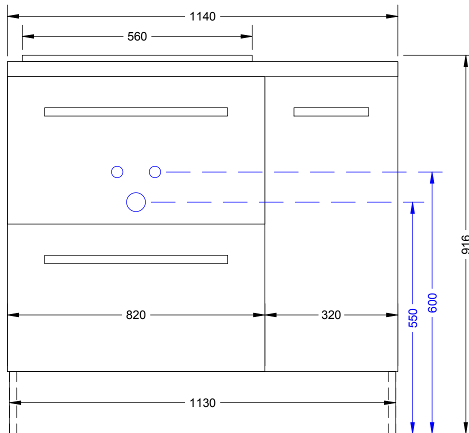
PŘEDNÍ POHLED
