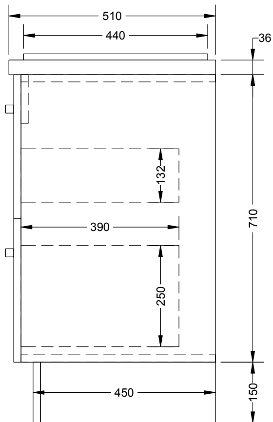
BOČNÍ POHLED
