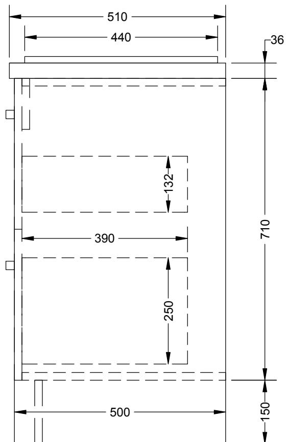
BOČNÍ POHLED
