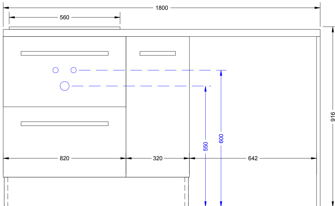
PŘEDNÍ POHLED
