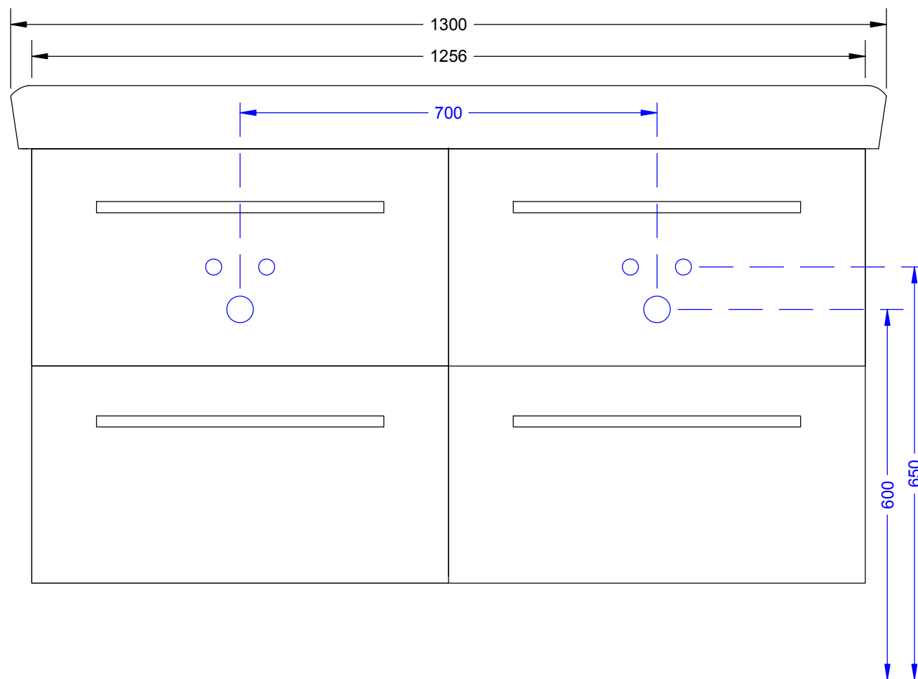
PŘEDNÍ POHLED
