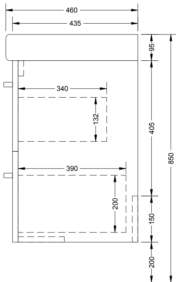
BOČNÍ POHLED
